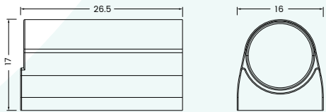
Sockel zur Unterbaumontage:
